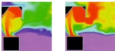
Fig.3 : Hotte à effet d'induction / Hotte d'extraction standard
